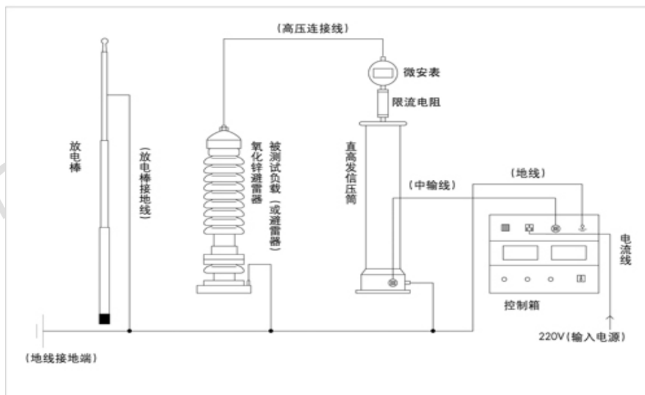
直流高压发生器线路图
